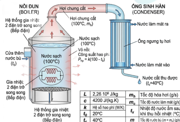
Hình 3: Sơ đồ hệ thống chưng cất có thu hồi nhiệt (mô hình dành cho ý 1)
