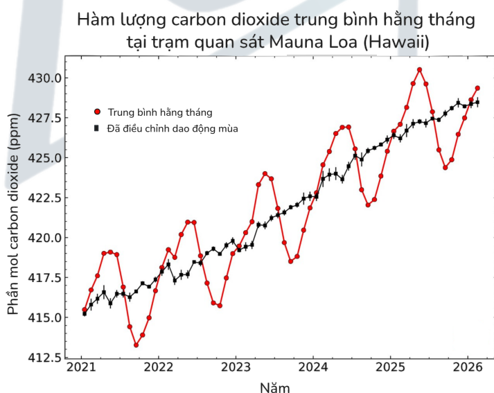
Hình 1: Nồng độ \text{CO}_2 (ppm) khí quyển trung bình hằng tháng tại trạm quan sát Mauna Loa (Hawaii) 1/2021-2/2026.
